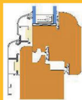
sezione infisso legno/alluminio
