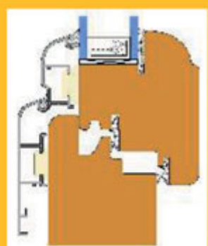
sezione infisso legno/alluminio
