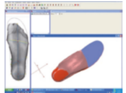
Elaborazione con il CAD di un PLANTARE
