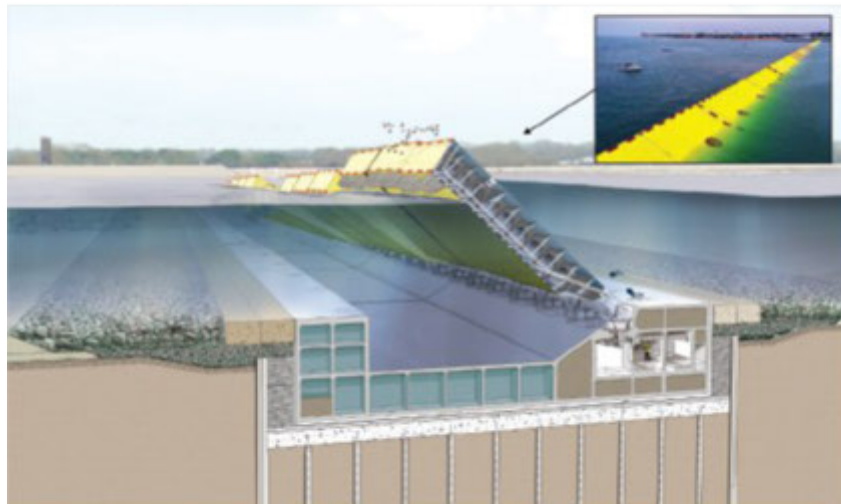
VI SONO QUATTRO BARRIERE Fisse POSTE ALLA FOCE DEL LIDO, DEL MALAMOCCO E DEL CHIOGGIA
